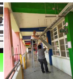
電力線槽施工
